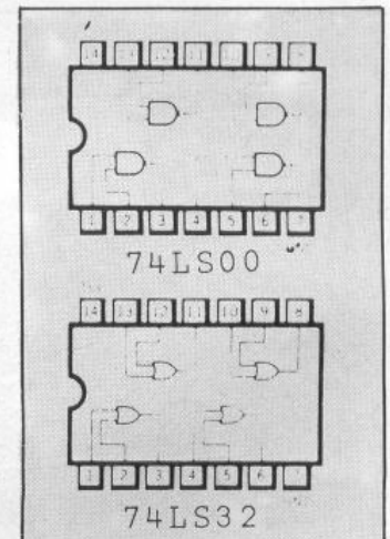
Descripción de patillaje. 74 LS 00 74 LS 32
